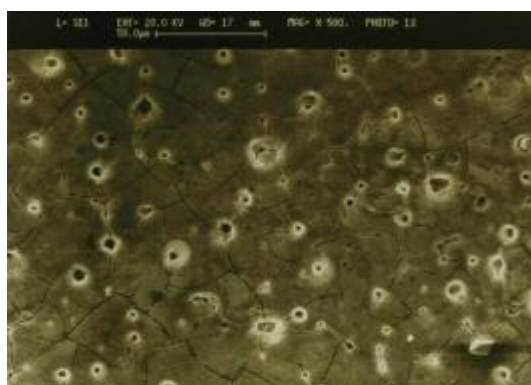
شکل ۹- تصویر میکروسکوپ الکترونی از سطح یک پوشش ترک دار حاصل از روش مستقیم بعد از آزمایش خوردگی دارای ترکیب آلیاژی Zn=70\% و Ni=30\%
