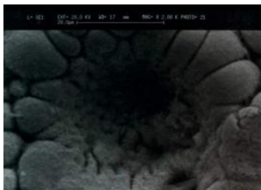
شکل ۸- سطح پوشش بعد از انجام آزمایش خوردگی راست) نمونه مستقیم با ترکیب آلیاژی Zn=52.8\% و Ni=47.2\% چپ) نمونه منقطع با ترکیب آلیاژی Zn=81.9\% و Ni=18.1\%
