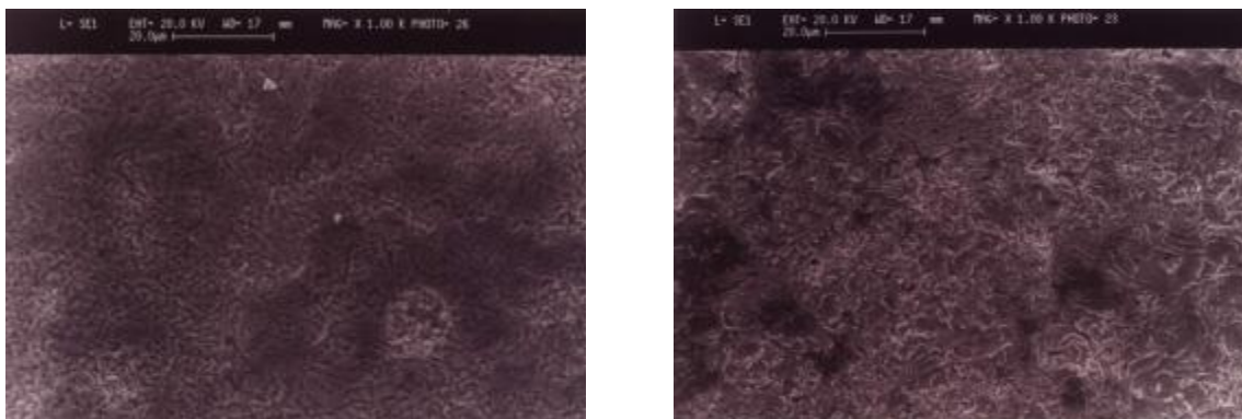
شکل ۴- تصویر SEM از سطح پوشش حاصل از روش منقطع با شرایط: راست) I_{peak} = 40 \text{ A/dm}^2 ; On-Time = ۱۰٪ ; f = 500 \text{ HZ} ; t_{on} = 0.5 \text{ m sec} ; On-Time = ۱۰٪ ; I_{peak} = 40 \text{ A/dm}^2 (چپ) f = 500 \text{ HZ} ; t_{on} = 1/2 \text{ m sec}
