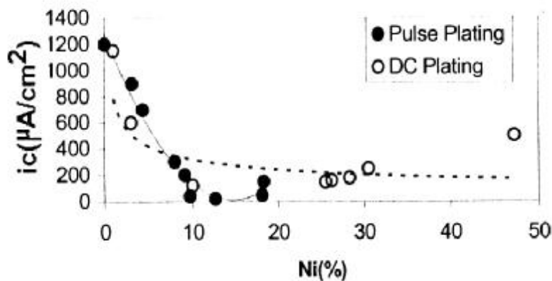
شکل ۷- تاثیر درصد نیکل در چگالی جریان خوردگی پوششهای آلیاژی روی- نیکل حاصل از آبکاری الکتریکی مستقیم و منقطع
