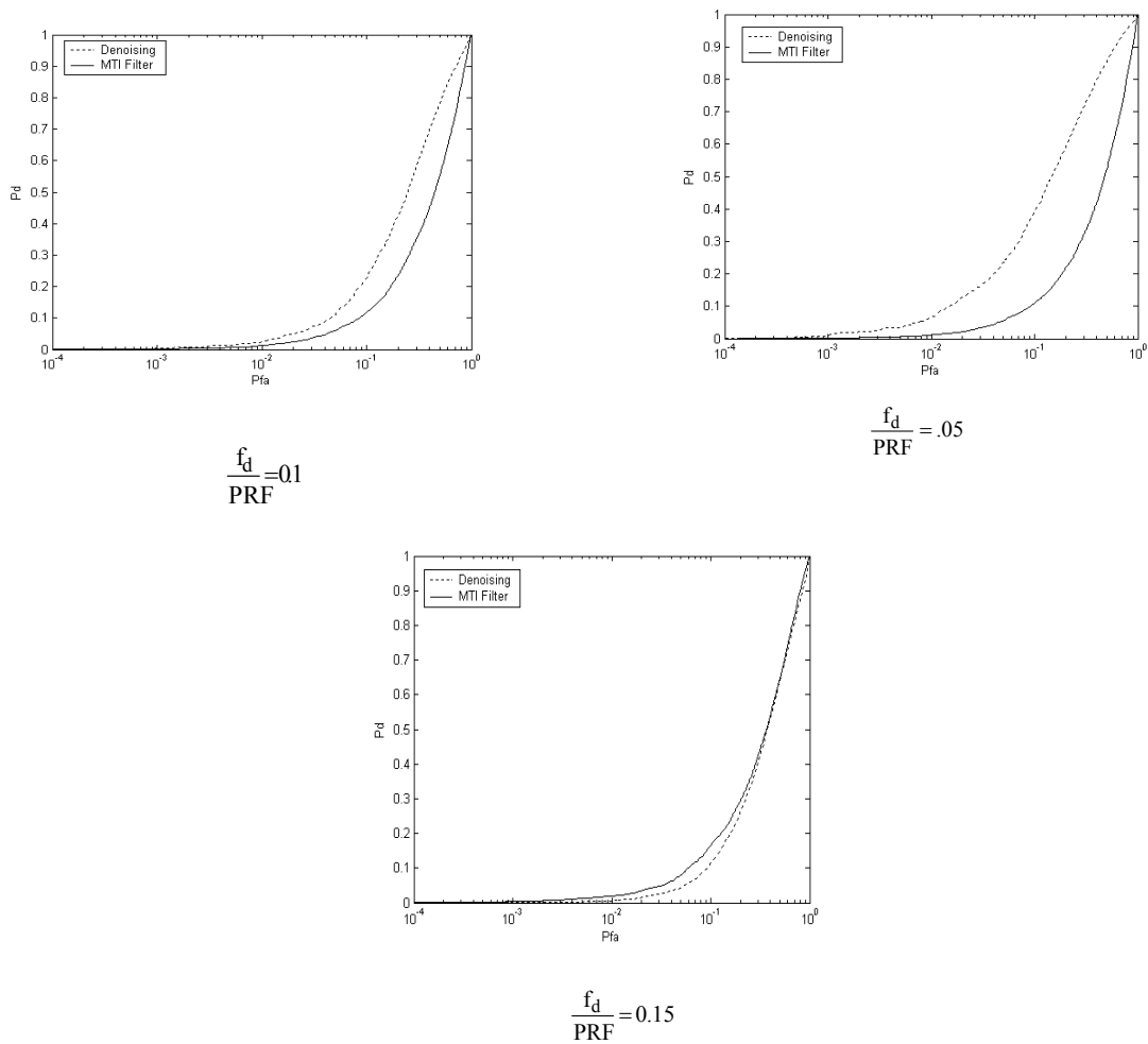
شکل ۹- منحنی احتمال آشکارسازی بر حسب احتمال آژیر غلط برای مقایسه کارایی فیلتر MTI و نویززدائی بر پایه تبدیل موجک
