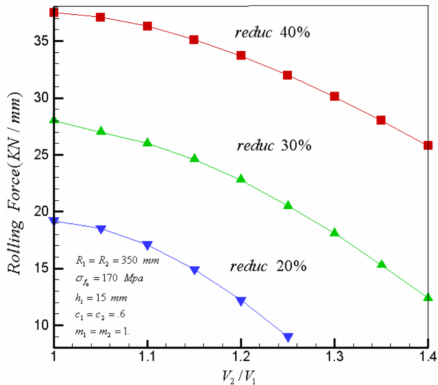
نمودار ۵- تغییرات نیروی نورد برحسب نسبت سرعتهای دو غلتک در کاهش ضخامتهای مختلف
