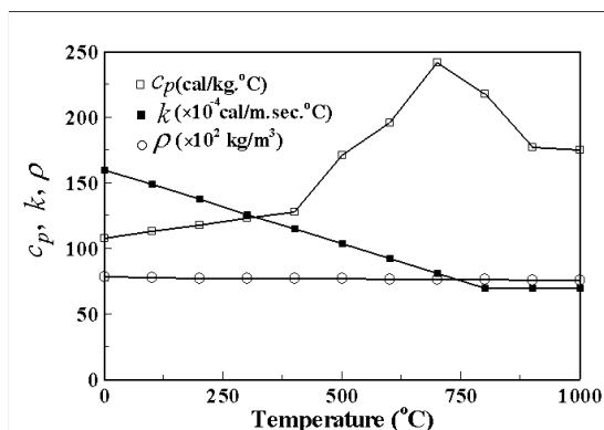
شکل ۷. خواص مکانیکی مواد به صورت تابع دما [۷]
