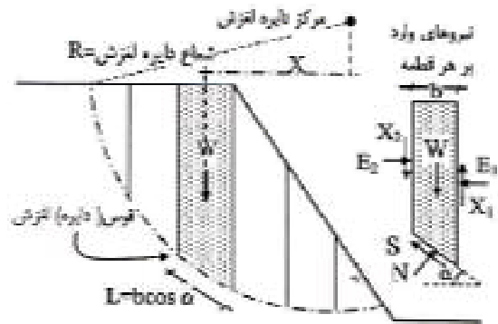
شکل ۱- سطح لغزش دایره‌ای آزمایشی در یک شیروانی در روش بیشاب
