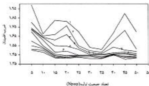
شکل ۱۰- تغییرات ضرب اطمینان در برابر تعداد جمعیت برای ۱۰ بار اجرای برنامه (مثال ۱)
