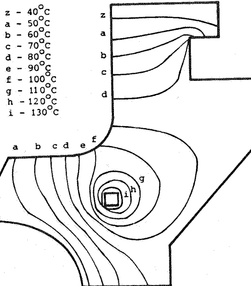
شکل ۲۱ - میدان دما در بدنه پمپ ( روش RIBEM )
