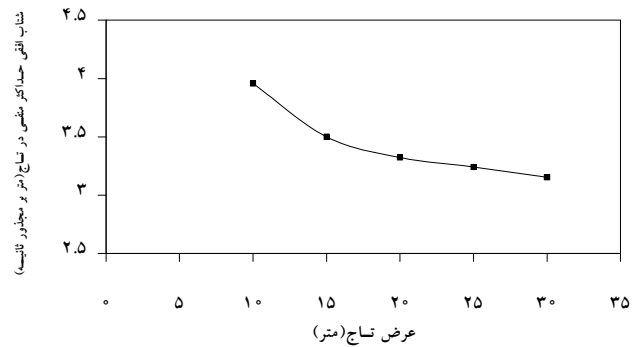
شکل ۳۸- رابطه شتاب حداکثر منتهی در تاج سد نسبت به عرض تاج سد برای زلزله "ناغان"
