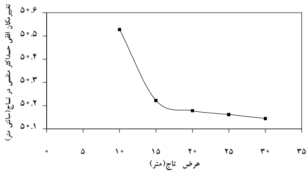
شکل ۳۹- رابطه جابه‌جایی افقی حداکثر منتهی در تاج سد نسبت به عرض تاج سد برای زلزله "ناغان"
