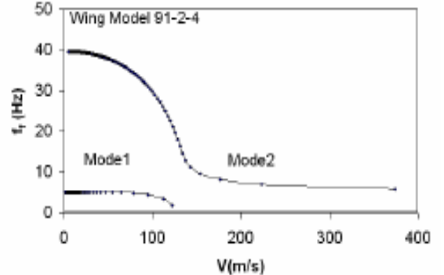
شکل ۷ - سرعت بر حسب فرکانس برای بال سری 91-2-4 حاصل از آزمایش تجربی [۲۲] و روش حاضر
