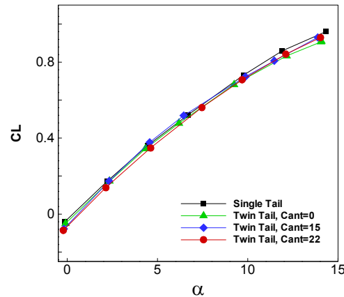
شکل ۶-الف) ضریب برآ در ماخ ۱/۴
