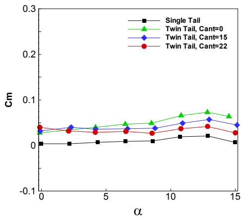
شکل ۵-د) ضریب گشتاور پیچشی
