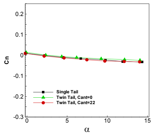
شکل ۷-ه) ضریب گشتاور جانبی در زاویه جانبی صفر درجه
