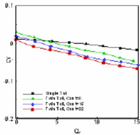
شکل ۵-ج) ضریب نیروی جانبی
