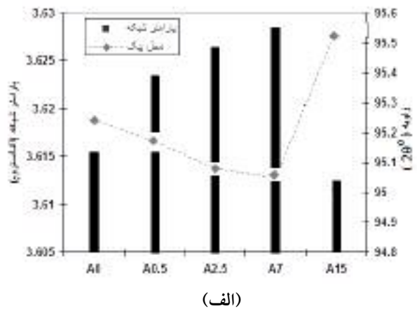
شکل ۲- تغییرات پارامتر شبکه و محل پیکها با پیشرفت آلیاژسازی مکانیکی الف) مس پیک (222). ب) نیکل پیک (311)
