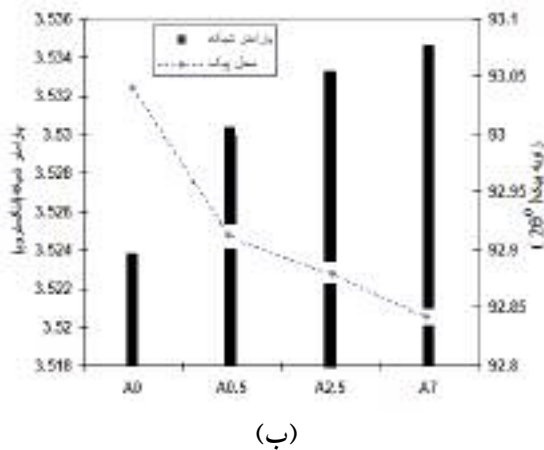
شکل ۲- تغییرات پارامتر شبکه و محل پیکها با پیشرفت آلیاژسازی مکانیکی الف) مس پیک (222). ب) نیکل پیک (311)
