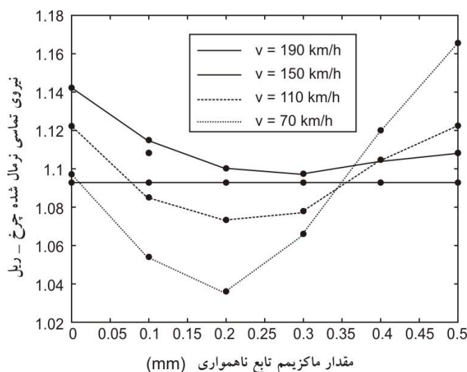
شکل ۱۴- بیشینه نیروی تماسی نرمال شده ریل - چرخ در ریل اصلی (نیروی تماسی استاتیکی نرمال شده) برحسب پارامتر ناهمواری A برای چهار سرعت مختلف وسیله نقلیه (۱۹۰، ۱۵۰، ۱۱۰، ۷۰) در مدل نیم بوژی
