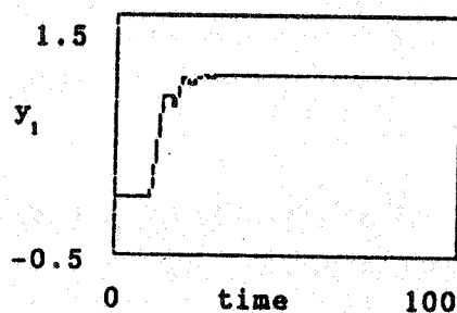
شکل ۱۱- پاسخ کنترل‌کننده‌های C و \bar{C} به ازاء یک تغییر پله‌ای در y_r برای مدل وود و بری با تأخیرهای اضافی و اعمال آنتی‌واین‌دآپ کمپو و موراری.
