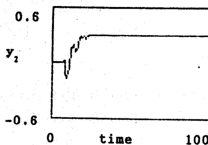
شکل ۱۱- پاسخ کنترل‌کننده‌های C و \bar{C} به ازاء یک تغییر پله‌ای در y_r برای مدل وود و بری با تأخیرهای اضافی و اعمال آنتی‌واین‌دآپ کمپو و موراری.
