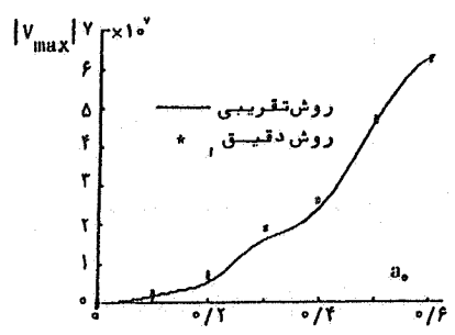
ج - حداکثر نیروی برشی
