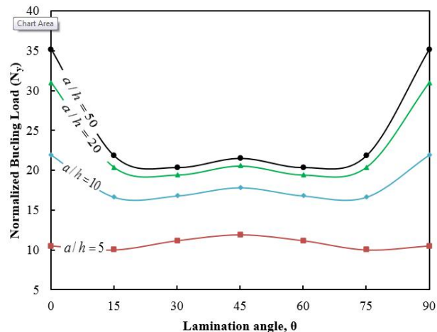
شکل ۶- ضربید بدون بعد کمانش در مقابل زوایای مختلف الیاف یک ورق چندلایه ارتوتروپیک مربعی با شرایط مرزی چهار طرف مفصل با ترکیب لایه [\theta^\circ / -\theta^\circ] برای نسبت بعد به ضخامت a/h مختلف و مدول الاستیسته E_1/E_2 = 40
