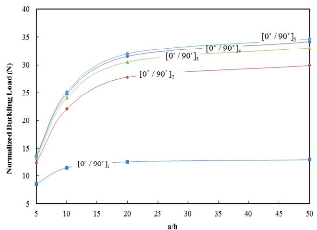
شکل ۴- ضریب بدون بعد کماتش در مقابل نسبت بعد به ضخامت a/h یک ورق چندلایه ارتوترپیک مربعی با شرایط مرزی چهار طرف مفصل با ترکیب لایه [0^\circ / 90^\circ]_n برای n = 1, 2, 3, 4, 5 بر حسب تعداد لایه‌ها با E_1 / E_2 = 40
