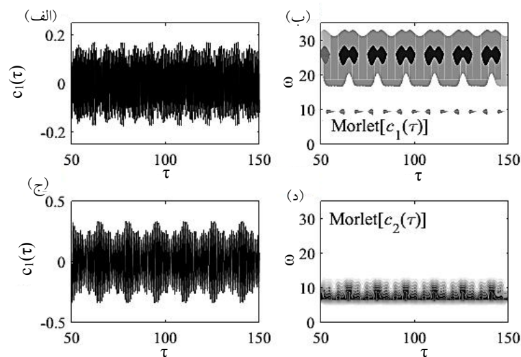
شکل ۹- الف) تابع مود ذاتی اول، ب) تبدیل موجک مورلت تابع مود ذاتی اول، ج) تابع مود ذاتی دوم و د) تبدیل موجک مورلت تابع مود ذاتی دوم از پاسخ زمانی ناپایدار به ازای \varepsilon\sigma_0 = 2/1
