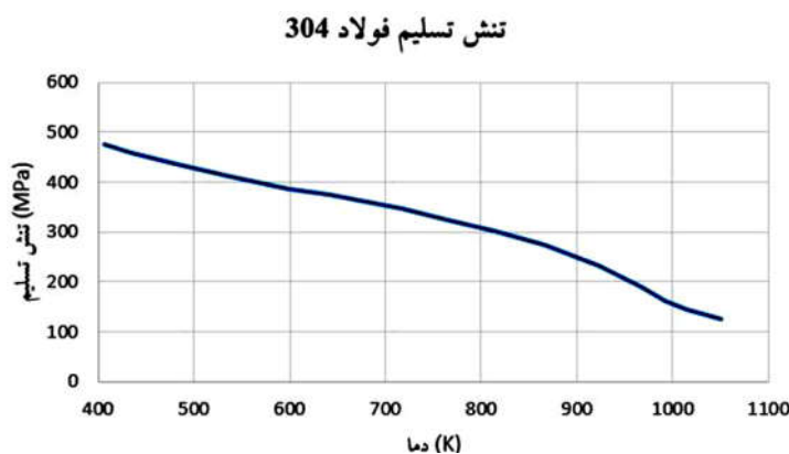
شکل ۶- تغییرات تنش تسلیم با دما برای فولاد زنگ‌نزن ۳۰۴ [۶]
