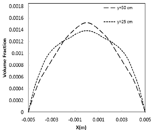
شکل ۹- توزیع کسر حجمی نانوذرات اکسید مس در ناحیه ابتدای کانال ( y = 25 cm) و انتهای کانال ( y = 50 cm) در یک
