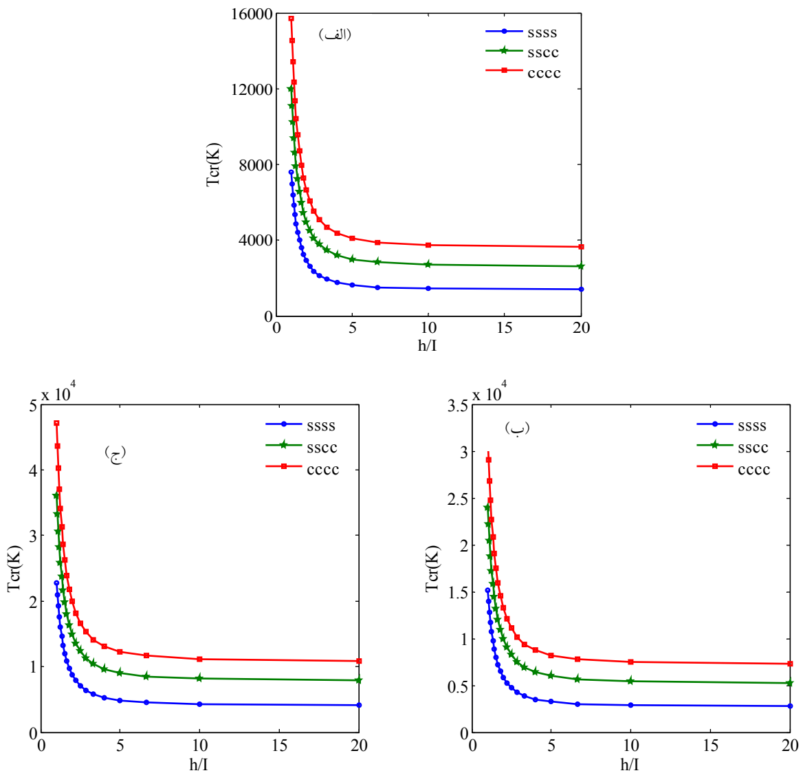
شکل ۵- نمودار تغییرات دمای بحرانی ورق مربعی برحسب نسبت ضخامت به پارامتر مقیاس طول
