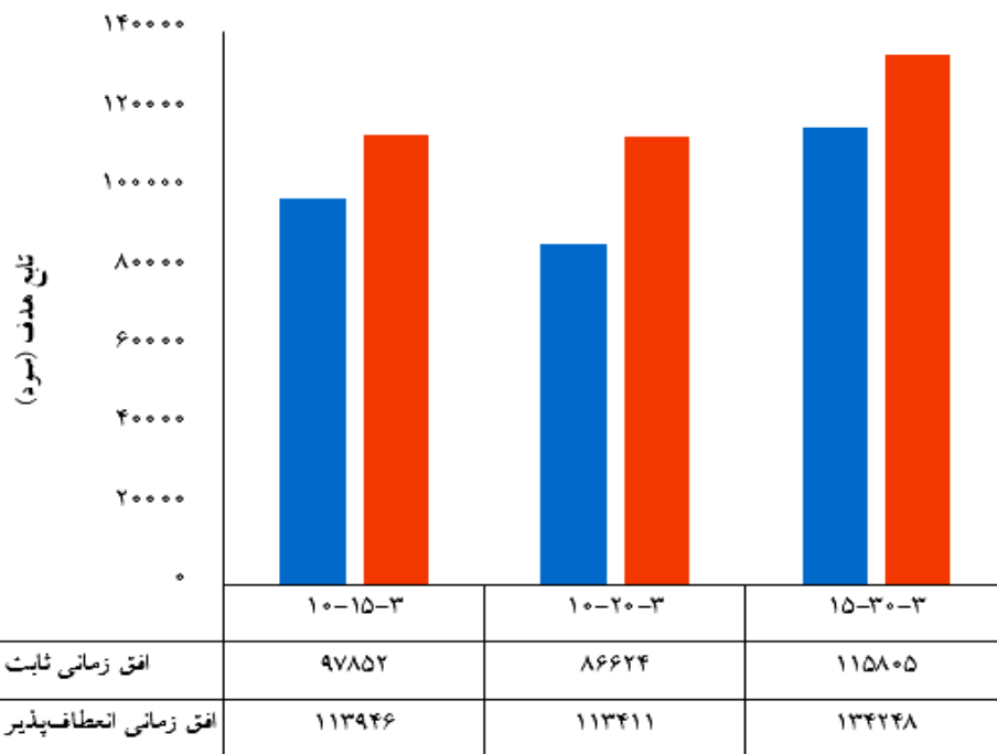
شکل ۱۶- میانگین مقادیر تابع هدف در دو حالت افق زمانی ثابت و انعطاف‌پذیر با الگوریتم ترکیبی ابتکاری پیشنهادی
