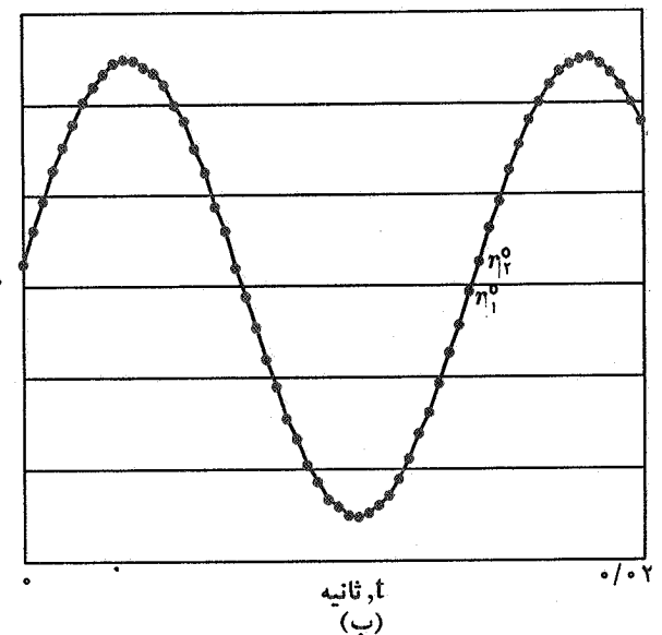
شکل ۵ - (الف) نتایج اندازه‌گیری سیم داغ در x = 35 cm و y = 0 ، (ب) مؤلفه زیرهماهنگ نمونه برداری شده سیگنال محرک که مفهوم نمونه برداری تطبیقی را برای تولید تصاویر مرکب نشان می‌دهد.
