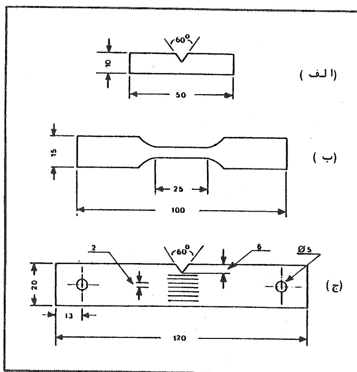
شکل ۱: انواع نمونه‌های مورد استفاده، ابعاد و مشخصات آنها.
