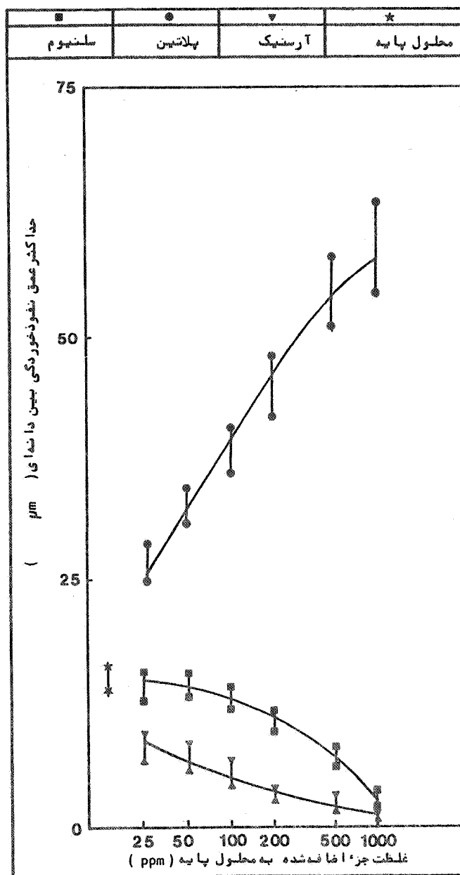
شکل ۱۲ : تأثیر غلظت سموم کاتدی مختلف در محلول پایه بر حداکثر عمق نفوذ خوردگی بین دانه‌ای ، زمان غوطه‌وری ۲۰ ساعت ،
