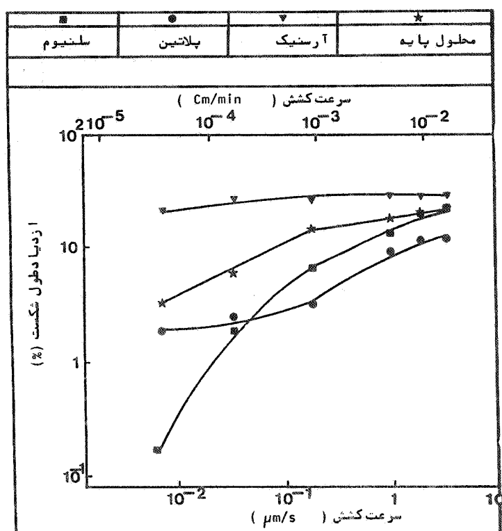
شکل ۷ : تأثیر سرعت کشش و نوع سموم کا تدی (غلظت 25ppm)
