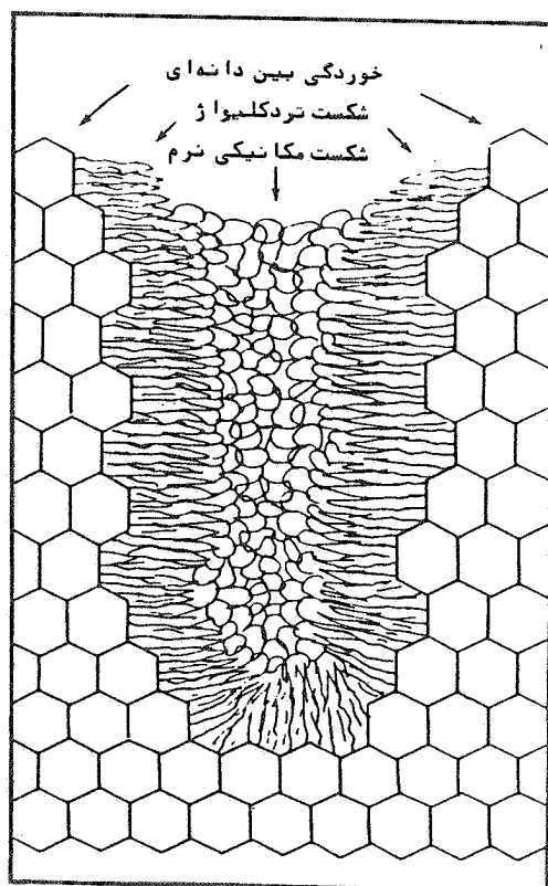
شکل ۱۳: نمایش شماتیک چگونگی توزیع و موقعیت نواحی خوردگی بین دانه‌ای، شکست مکانیکی نرم و شکست تردکلیواژ بر روی سطوح مقطع شکست نمونه‌های آزمایش شده تحت شرایط خوردگی تنشی.
