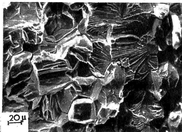
شکل ۱۴ : تصویر میکروسکوپی الکترونی از سطح مقطع شکست شامل سه ناحیه خوردگی بین دانه‌ای ، شکست ترد کلیواژ و شکست نرم مکانیکی ، محلول مورد استفاده : محلول پایه سرعت کشش : 3/3 \times 10^{-1} میکرون بر ثانیه
