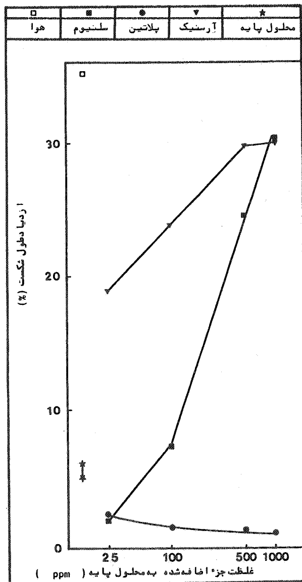
شکل ۴ : تا شیر غلظت سموم کا تدی اضافه شده با محلول پایه برگزینش شکست. سرعت کشش : 2/3 \times 10^{-2} میکرون بر ثانیه
