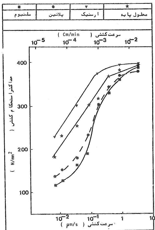
شکل ۶: تاثیر سرعت کشش و نوع سموم کاتدی (غلظت 25ppm) اضافه شده به محلول پایه بر استحکام کششی
