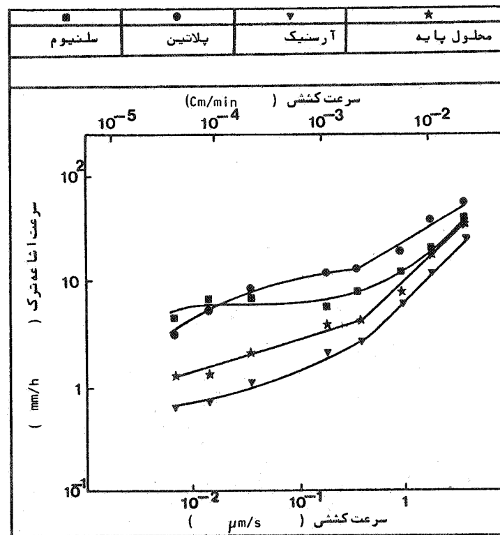
شکل ۸ : تأثیر سرعت کشش و نوع سموم کا تدی ( غلظت 25 ppm ) اضافه شده به محلول پایه بر سرعت اشاعه ترک .
