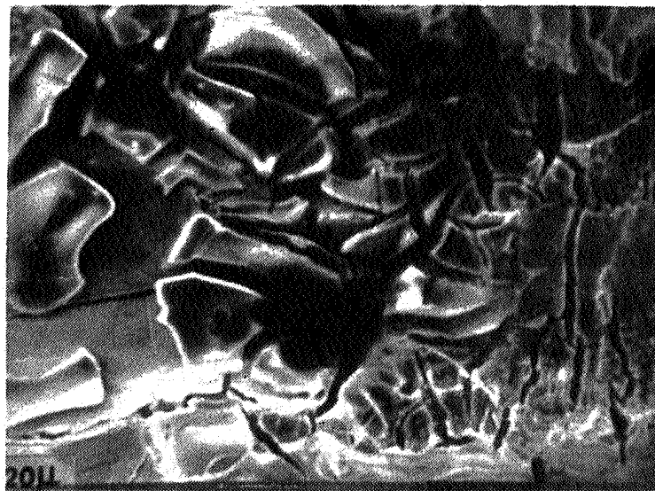
شکل ۱۶ : تصویر میکروسکوپی الکترونی از رسوبات غنی از پلاتین تشکیل شده بر روی سطوح نمونه های خوردگی تنشی. محلول، محلول پایه حاوی 1000ppm پلاتین. سرعت کشش ، 8/3 \times 10^{-3} میکرون بر ثانیه .
