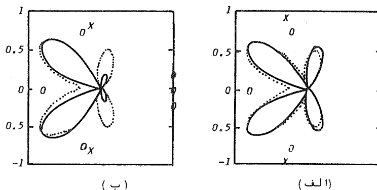
شکل ۱۵ : پاسخهای فرکانسی فیلترهای حذف‌کننده نمونه همراه با مکان صفرهای آنها در صفحه Z (الف) تاثیر تغییر اندازه صفرها بر پاسخ فرکانسی (ب) تاثیر تغییر زاویه صفرها بر پاسخ فرکانسی
