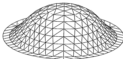
شکل ۳- شبکه بندی مورد استفاده در اتساع متقارن محوری
