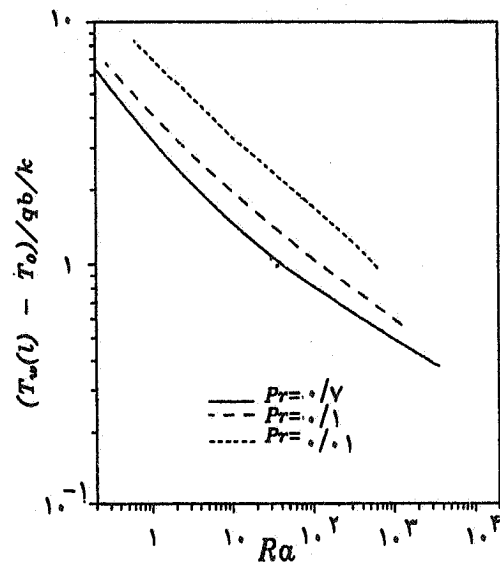
شکل ۱۴ - تغییرات ماکزیمم دمای سطح بر حسب عدد رایلی
