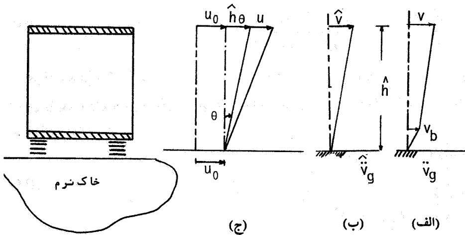
شکل ۴ - مراحل متوالی تعیین سیستم معادل یک درجه‌آزادی
