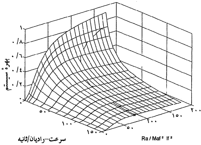
شکل ۲۲- بهره سیستم در موتور تحریک جداگانگانو حداکثر آن در سرعت ثابت: -
