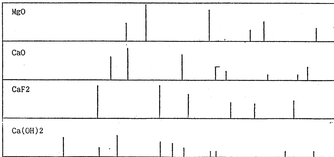
شکل ۲- قله‌های فازهای انتخاب شده برای آجر نسوز دولومیتی منیزیتی هیدراته شده
