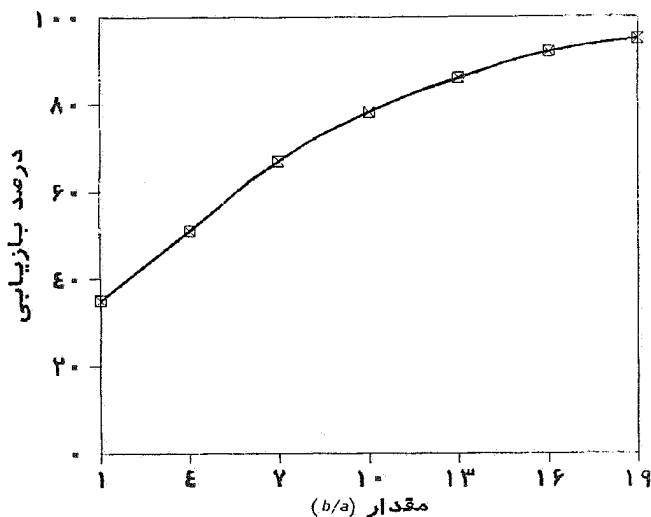
شکل ۱۳- تاثیر میزان سود مصرفی بر بازیابی وانادیم در دمای 90^\circ\text{C} (نسبت مولی \text{NaOH} به \text{V}_2\text{O}_5 است)
