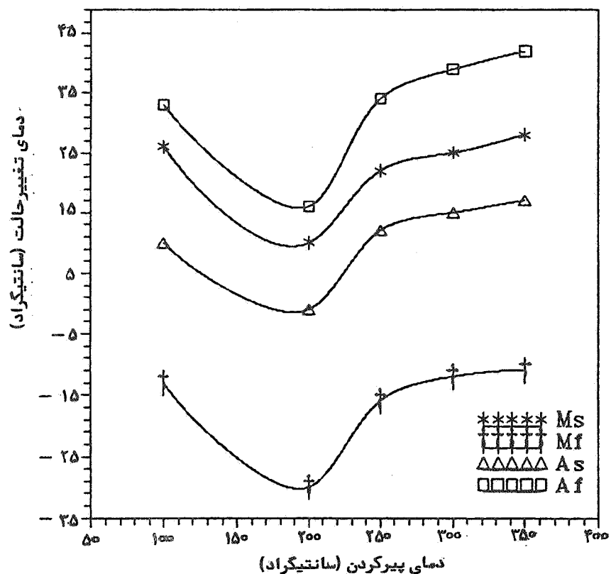
شکل ۹ - تأثیر دمای پير کردن بر دماهای تغيير حالت
