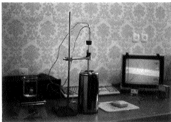
شکل ۴ - دستگاه اندازه گیر مقاومت الکتریکی بر حسب دما
