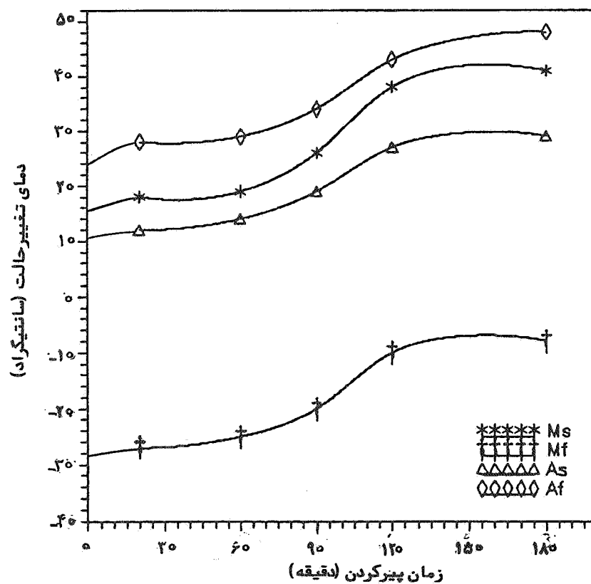
شکل ۱۰ - تأثیر زمان پير کردن بر دماهای تغيير حالت
