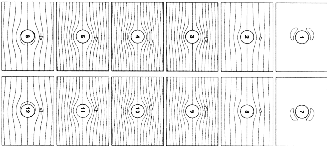
شکل ۱- از راست به چپ به ترتیب خطوط وزیستی و خطوط جریان برای حالت‌های استوانه نوسانی و جریان نوسانی به ازای KC = 1.0 ، \beta = 35
