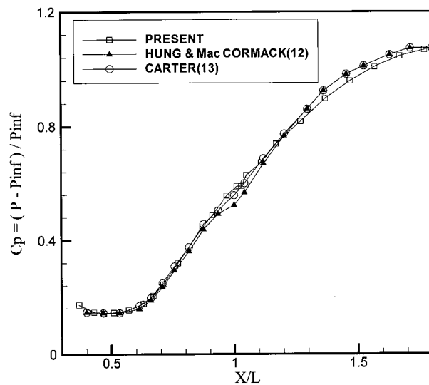
شکل ۵- مقایسه توزیع فشار روی سطح با نتایج عددی برای M=3
