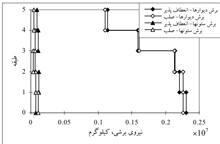
شکل ۸- مقایسه نیروی برشی دیوارها، ستونها و طبقه در تحلیل سازه با فرض دیوارهای صلب و انعطاف پذیر، نمونه ۲
