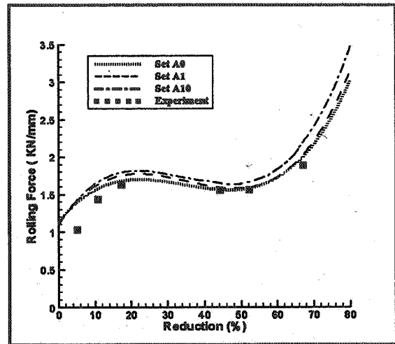
شکل ۱۲- نیروی نورد
