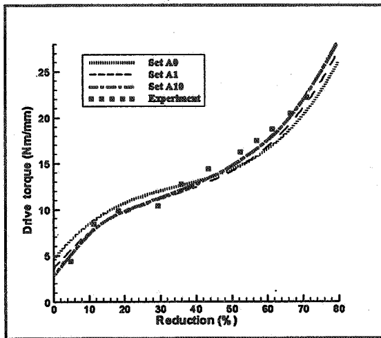
شکل ۱۳- گشتاور نورد
