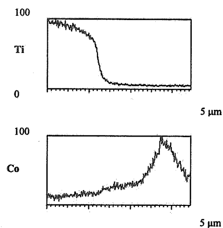
شکل ۵- میکروگراف الکترونی همراه با آنالیز خطی در موضع اتصال جوش اصطکاکی Ti6Al4V/WC-24 wt.%Co
