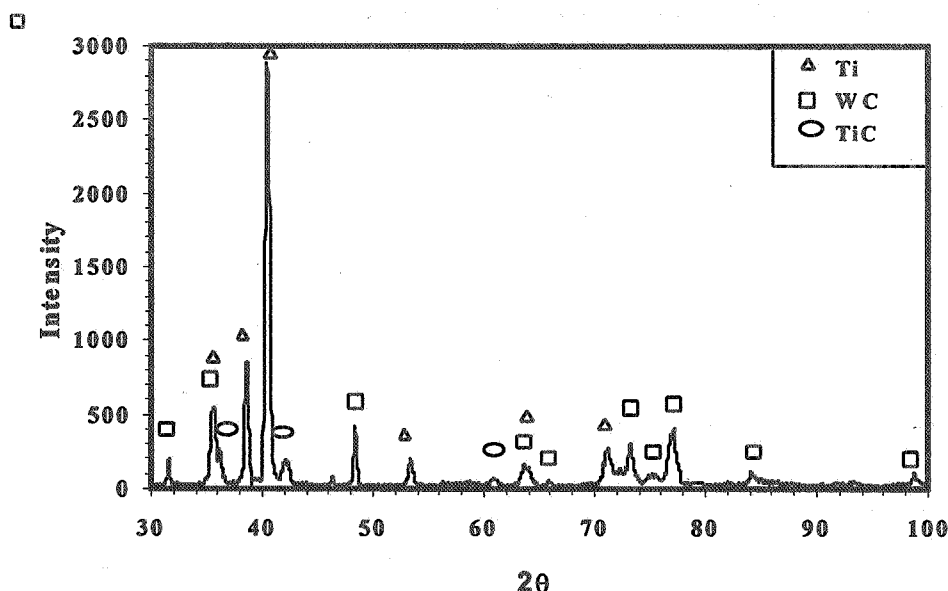
شکل ۷- آزمایش پراش پرتو ایکس (XRD) بر سطح مقطع شکست جوش اصطکاکی Ti6Al4V/WC-11 \text{ wt.\%Co} (در سمت تیتانیم)
