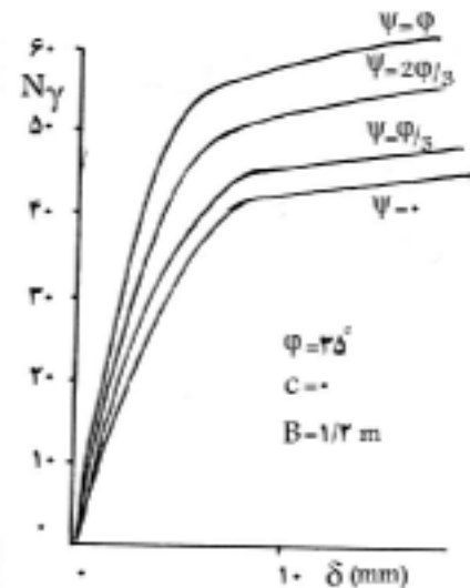
شکل ۶- نمونه‌ای از چگونگی اثر افزایش زاویه اتساع بر مقدار نهایی ظرفیت باربری
