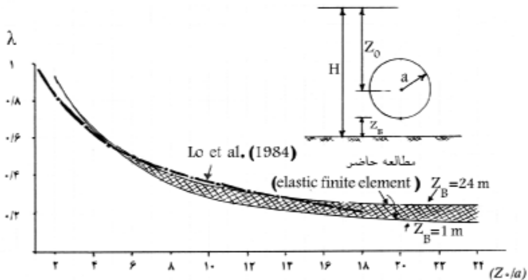
شکل ۱۵- تغییرات (\lambda) بر حسب z_0/a برای شرایط Z_B=1\text{ m} و 24\text{ m} در محاسبات حاضر (\nu=0)
