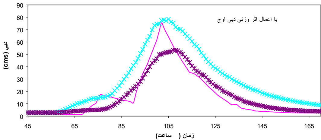
شکل ۱۲- محدوده پیش بینیها با اثر یکسان و اثر وزنی دبی هیدروگراف سیلاب مورخ ۱۸ آذر ۵۷
