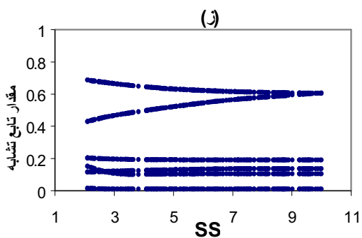
شکل ۷- حساسیت تابع تشابه معادله ۱۰ با N=1 نسبت به تغییرات پارامترهای نفوذ نمایی، R و TC (الف- پارامتر زمان تمرکز، ب- پارامتر ضریب ذخیره، ج- پارامتر نفوذ اولیه باران SR، د- پارامتر DL نفوذ باران، هـ) پارامتر RL نفوذ باران، و- پارامتر ER نفوذ باران، ز- پارامتر SS نفوذ ذوب برف و ح- پارامتر RK نفوذ ذوب برف)
