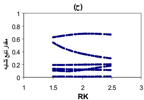
شکل ۷- حساسیت تابع تشابه معادله ۱۰ با N=1 نسبت به تغییرات پارامترهای نفوذ نمایی، R و TC (الف- پارامتر زمان تمرکز، ب- پارامتر ضریب ذخیره، ج- پارامتر نفوذ اولیه باران SR، د- پارامتر DL نفوذ باران، هـ) پارامتر RL نفوذ باران، و- پارامتر ER نفوذ باران، ز- پارامتر SS نفوذ ذوب برف و ح- پارامتر RK نفوذ ذوب برف)
