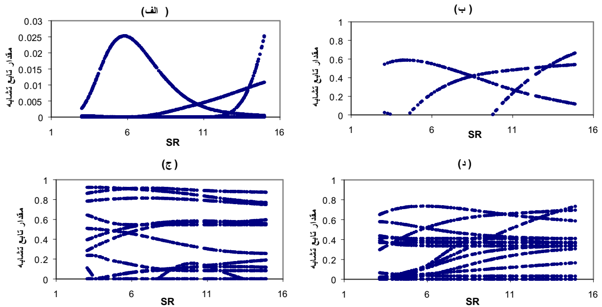
شکل ۹- پراکندگی معیارهای تشابه مختلف نسبت به پارامتر SR (الف- تابع معادله ۱۰ با N=10 ، ب- تابع تشابه وزنی، ج- تابع لگاریتم داده ها، د- تابع رابطه ۱۴ با N=14 )
