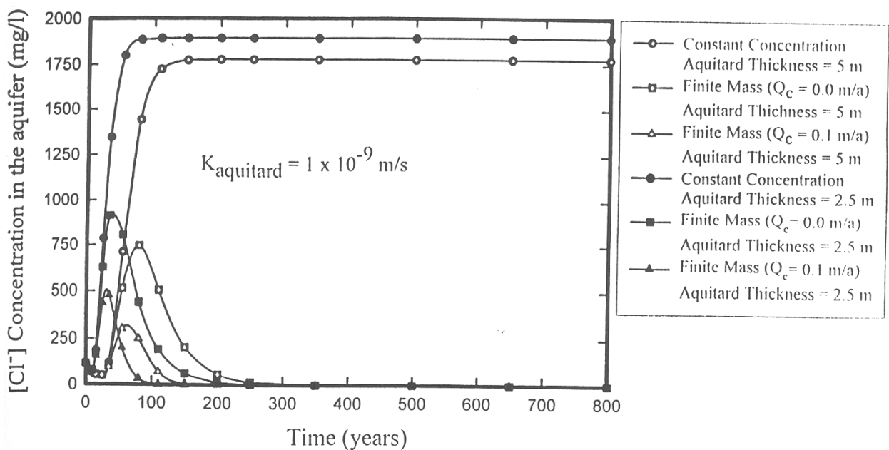
شکل ۸ - تغییرات غلظت یون کلر (Cl) در سفره آبدار نسبت به زمان در مدفن زباله با زهکشهای فرانسوی (گزینه دوم) در حالت طبیعی، (۱) تاثیر غلظت ثابت نسبت به غلظت یا جرم محدود در کف مدفن، (۲) تاثیر ضخامت لایه زمین طبیعی، K_{aquitard} = 1 \times 10^{-9} (m/s)، (۳) تاثیر میزان زهکشی شیرابه در کف مدفن.
