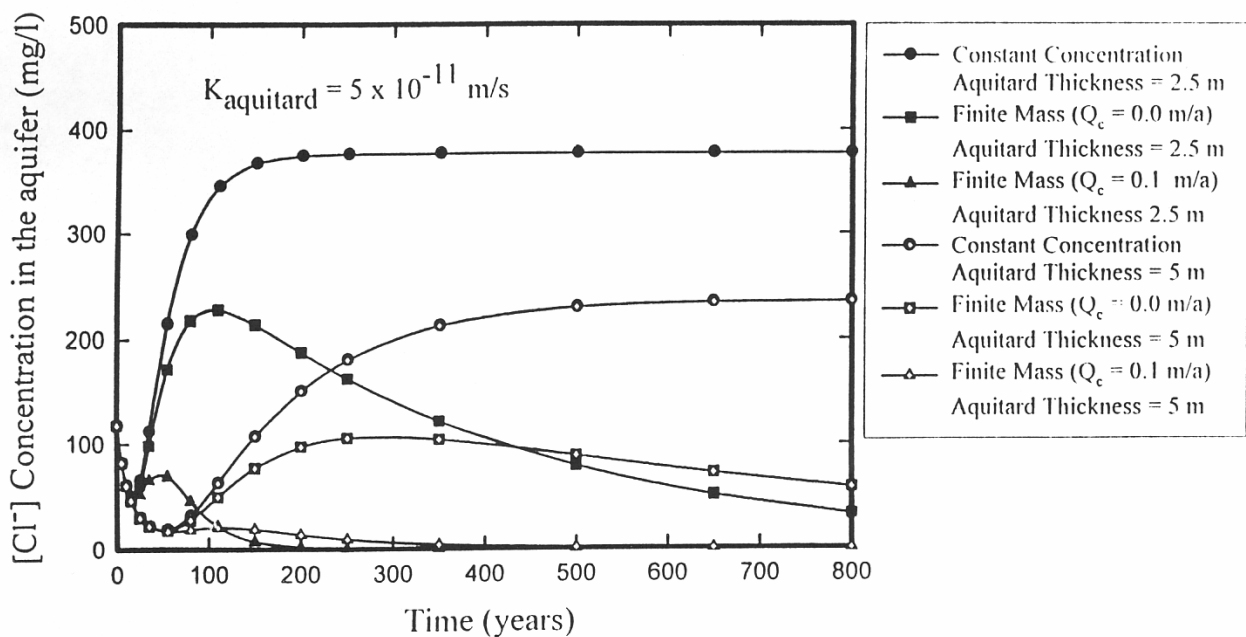
شکل ۷ - تغییرات غلظت یون کلر (Cl) در سفره آبدار نسبت به زمان در مدفن زباله با زهکشهای فرانسوی (گزینه دوم) در حالت طبیعی، (۱) تاثیر غلظت ثابت نسبت به غلظت یا جرم محدود در کف مدفن، (۲) تاثیر ضخامت لایه زمین طبیعی، K_{aquitard} = 5 \times 10^{-11} (m/s)، (۳) تاثیر میزان زهکشی شیرابه در کف مدفن.
