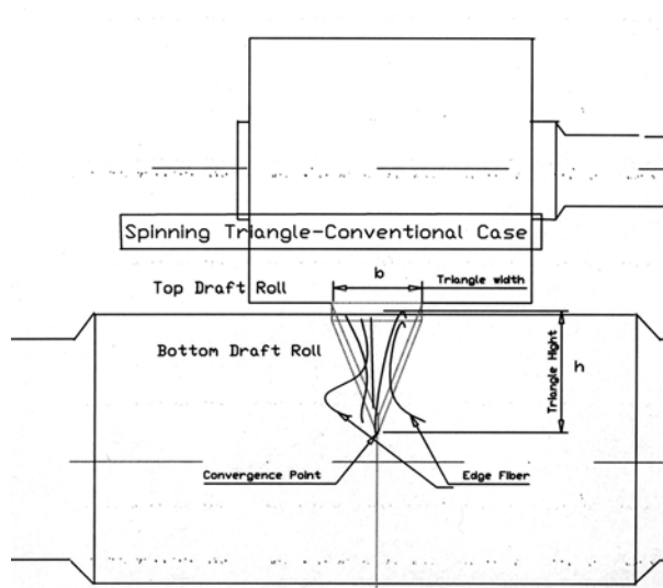
شکل ۴ - هندسه مثلث ریسندگی در حالات معمولی و تغییر شکل یافته
