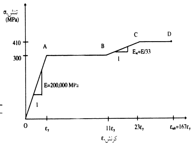
شکل ۴- منحنی تنش - کرنش ایدئال شده فولاد [۸]
