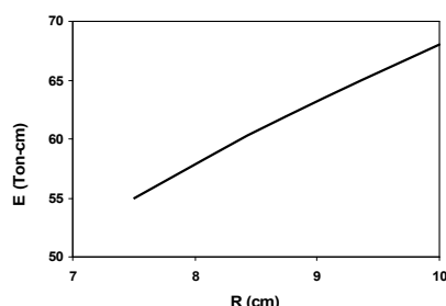
شکل ۱۹- تأثیر ضخامت جداره بر اتلاف انرژی لوله آکاردئونی با جداره دایره‌ای شکل
