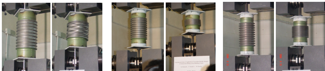
شکل ۷- تغییر شکل فشاری و کششی محوری در آزمایش دینامیکی لوله‌های جدار نازک آکاردئونی
