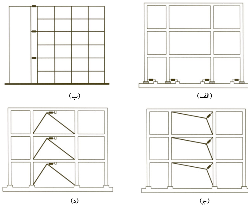
شکل ۲۵- کاربرد میراگر فلزی آکاردئونی در مقاوم سازی لرزه‌ای قابها و موقعیت قرارگیری آنها
