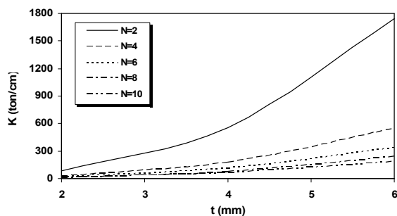
شکل ۱۶- تأثیر تعداد پلیس‌ها و شعاع لوله بر سختی الاستیک لوله جدار نازک آکاردئونی با جداره دایره ای شکل
