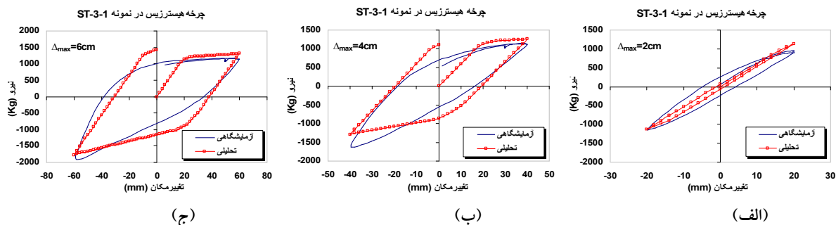
شکل ۱۰- مقایسه رفتار هیسترتیک در مطالعات آزمایشگاهی و تحلیلی در نمونه ST-1-3 در یک چرخه کامل بارگذاری (الف) دامنه تغییر مکان ۲ سانتیمتر ، (ب) دامنه تغییر مکان ۴ سانتیمتر، (ج) دامنه تغییر مکان ۶ سانتیمتر
