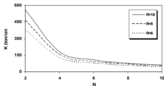
شکل ۱۵- تأثیر ضخامت و تعداد پلیس‌ها در سختی الاستیک لوله جدار نازک با جداره دایره‌ای شکل
