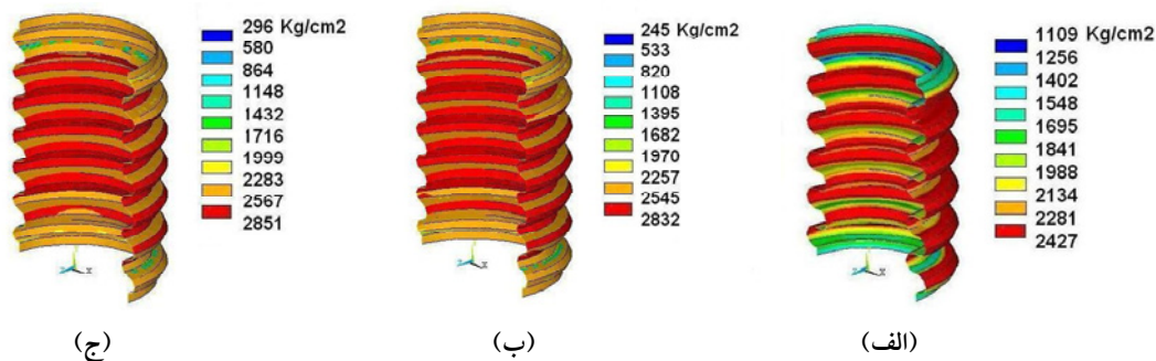
شکل ۱۳- وضعیت تنش در جداره لوله‌های جدار نازک آکاردئونی براساس معیار ون میس
