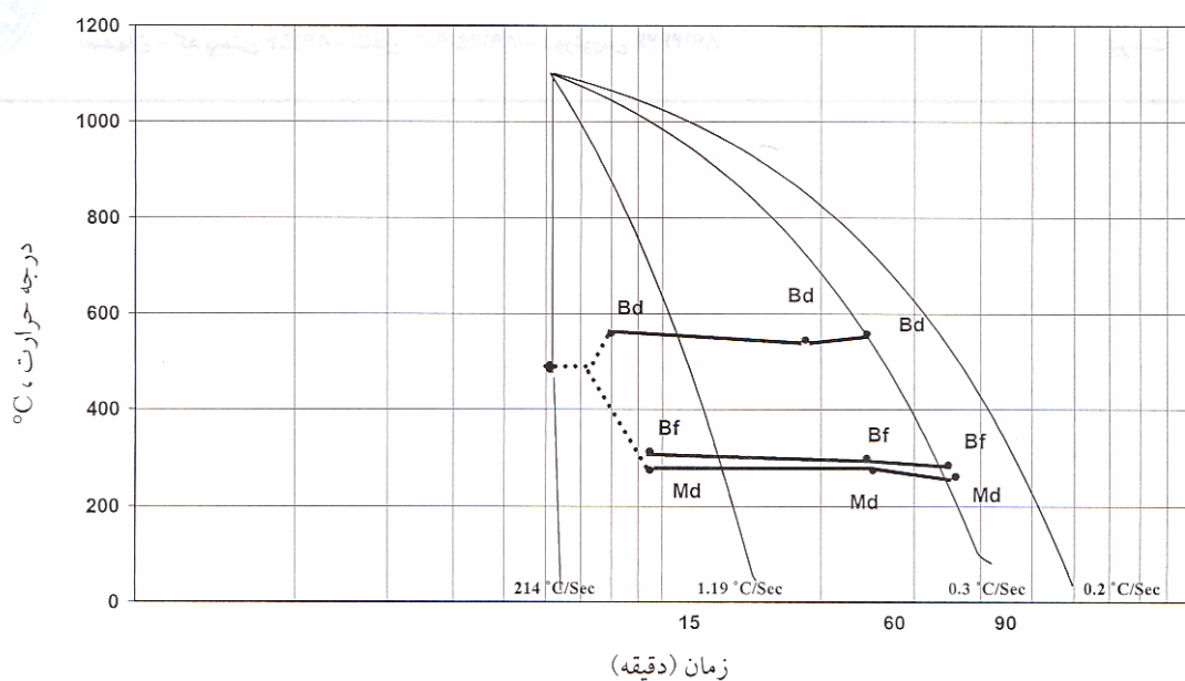
شکل ۲- نمودار CCCT فولاد NiCrMoV در حالت یک مرحله کرنش روی آستنیت اولیه در دمای 1100^{\circ}\text{C} ، با نرخ کرنش 0.1 \text{ s}^{-1} و کرنش 0.92 ، به معنای بینایت و M، به معنای مارتنزیت است نقاط نقطه چین، نقاط آزمایش نشده احتمالی را نشان می‌دهد
