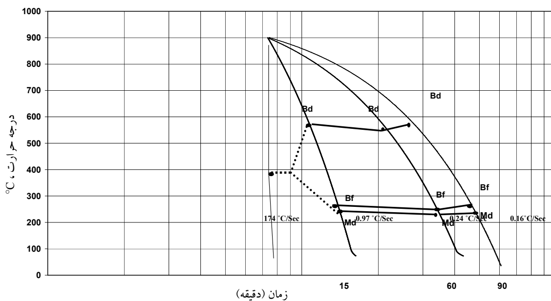
شکل ۳- نمودار CCCT فولاد NiCrMoV در حالت یک مرحله کرنش روی آستنیت اولیه در دمای 900^{\circ}\text{C} ، با نرخ کرنش 0.1 \text{ s}^{-1} و کرنش 0.92 ، به معنای بینایت و M، به معنای مارتنزیت است نقاط نقطه چین، نقاط آزمایش نشده احتمالی را نشان می‌دهد
