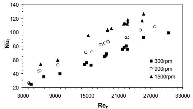
شکل ۱۰ - تغییرات عدد ناسلت متوسط روتور بر حسب عدد رینولدز محوری با دورهای مختلف
