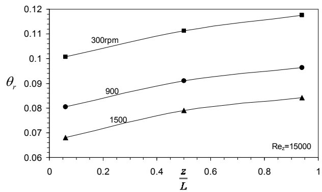
شکل ۸ - تغییرات محوری دمای سطح روتور در رینولدز ۱۵۰۰۰ با دورهای مختلف
