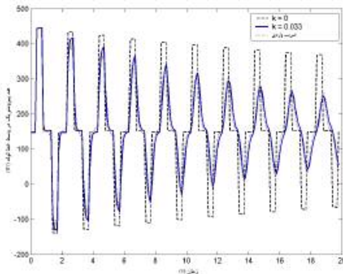
شکل ۸- مقایسه مقادیر مختلف ضریب k در مدل برونون با ضریب واردی در هد وسط لوله (قانون بستن شیر به صورت لوله) k = 0 به معنی عدم اعمال جمله اصطکاک ناماناست
