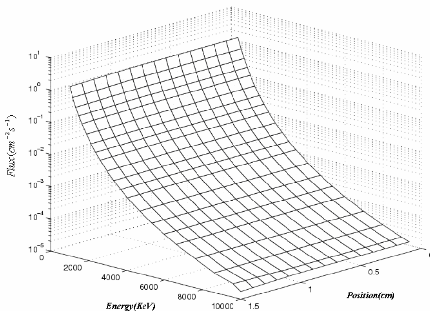
شکل ۱۲- شار الکترونیهای 1-10 MeV درون محیط سوخت در حضور میدان مغناطیسی (معادله فاکر پلانک)
