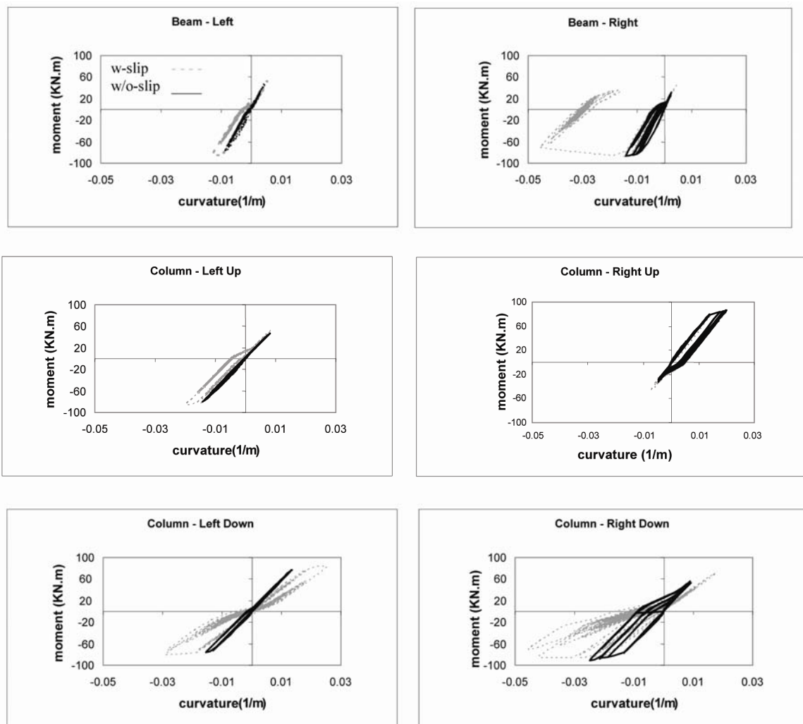
شکل ۹- منحنیهای ممان-انحنای برای حالت با و بدون لغزش
