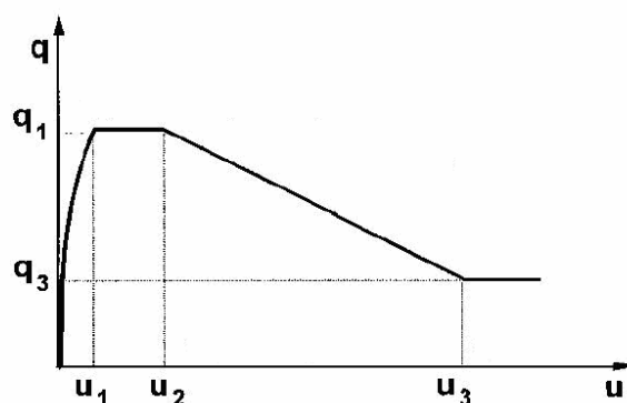
شکل ۱- منحنی تنش پیوستگی-لغزش پیشنهادی الیگهاوسن و همکاران
