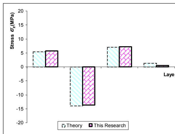
شکل ۶- مقایسه نتایج تحلیلی و تجربی مولفه تنش \sigma_x در هر لایه از چند لایه‌های [0_4 / 90_4]
