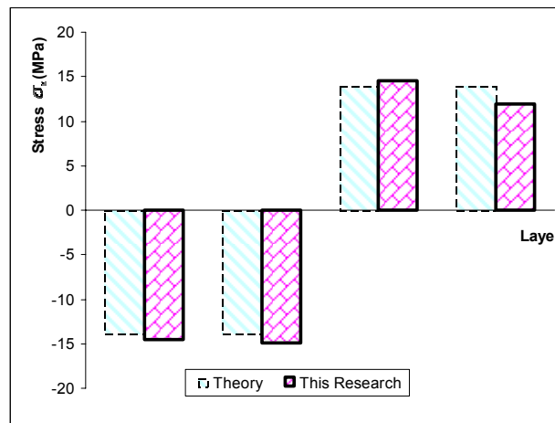
شکل ۴- مقایسه نتایج تحلیلی و تجربی مولفه تنش \sigma_x در هر لایه از چند لایه‌های [0_2/90_2]_S
