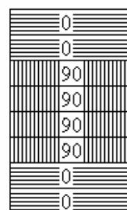
شکل ۲- الف) چیدمان متقارن چندلایه متعامد [0_2 / 90_2]_S
