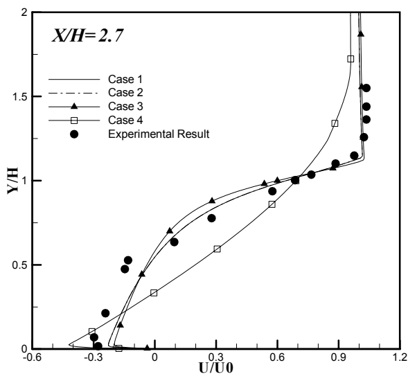
شکل ۷- مقایسه توزیعهای مؤلفه افقی سرعت در دو مقطع پایین دست پله برای
