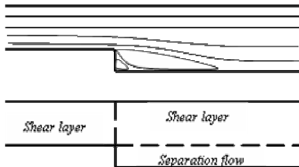
شکل ۳- پیش بینی خطوط جریان و مکانیزمهای اغتشاشی در مناطق مختلف میدان جریان
