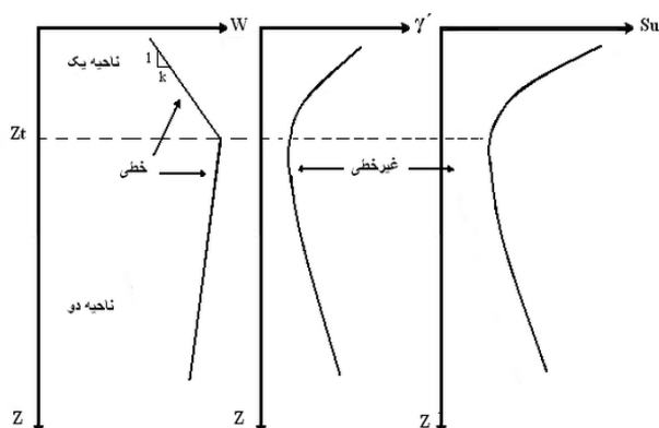
شکل ۱۱ - نمایش شماتیک تغییرات w ، \gamma' و S_u با عمق
