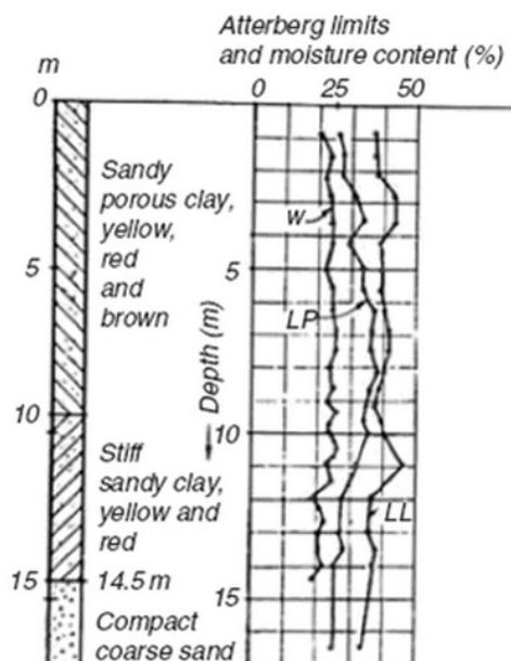
شکل ۷ - حدود اتربرگ و درصد رطوبت رس کامپیناس در برزیل [۳۲]
