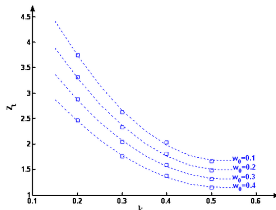
شکل ۱۲ - تأثیر در صد رطوبت سطحی ( w_0 ) و نرخ تغییرات در صد رطوبت با عمق ( k ) بر عمق تبدیل ( Z_t )
